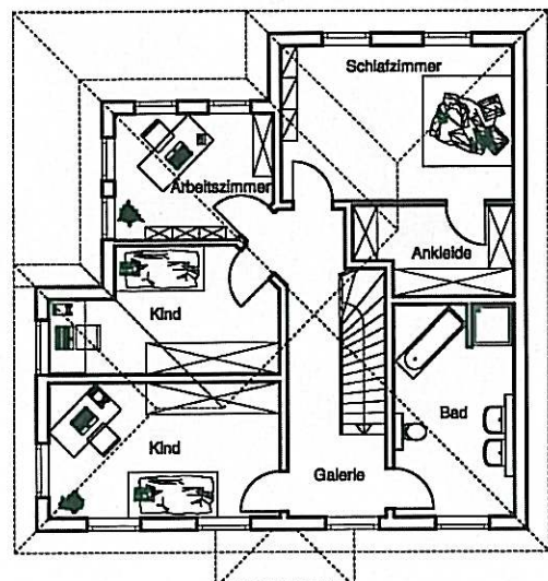
Grundriss Dachgeschoss
